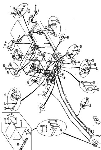
エレキトリカル システム Fig. 131A ELECTRICAL SYSTEM (1/2) (適用 車 種 Serial No. 1336~4000)
