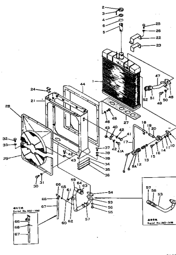
ラジエーター (適用 車 種 .....) Fig. 111 RADIATOR (Serial No. 1003~4000)
