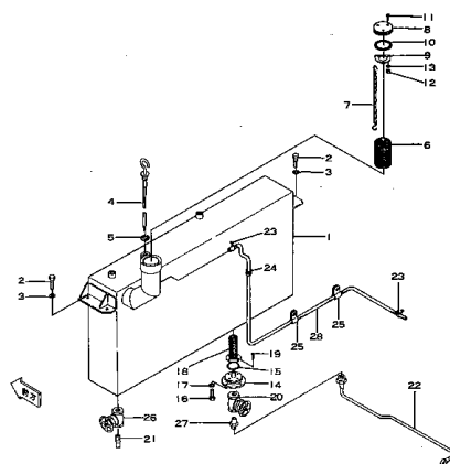
Fig. 112 FUEL TANK (適用 機種 Serial No. 1003~1335)
