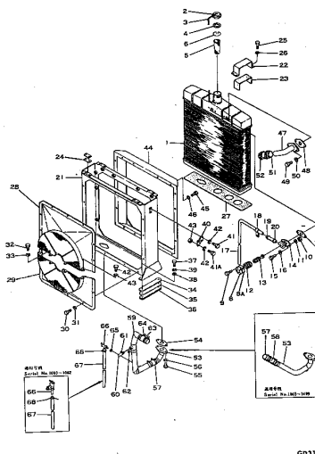
ラジエータ (適用車種: ...) Fig. 111 RADIATOR (Serial No. 1003~4000)
