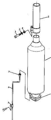
エキゾースト マフラー (適用号機) Fig. 102 EXHAUST MUFFLER (Serial No. 1003~1500)
