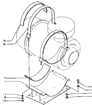
Fig. 101 AIR CLEANER MOUNTING (適用号数 Serial No. 1003~1499)
