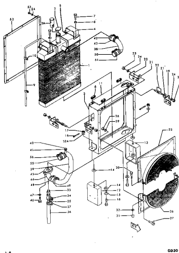
Fig. 113 RADIATOR
