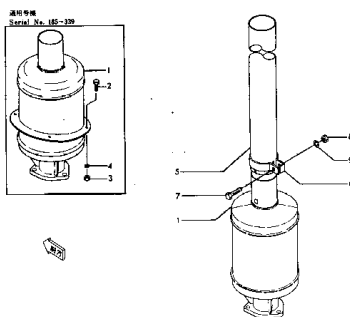
エキゾースト マフラー (適用号機) Fig. 112 EXHAUST MUFFLER (Serial No. 185~800)
