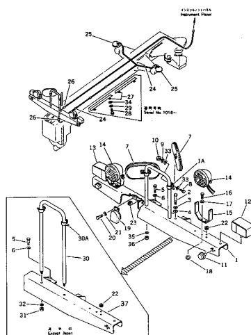
フロント エレクトリカル パーツ Fig. 141 FRONT ELECTRICAL PARTS
