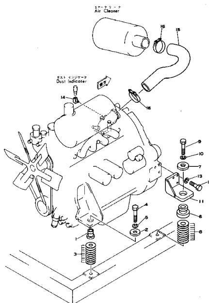
エンジン マウンティング パーツ Fig. 101 ENGINE MOUNTING PARTS
