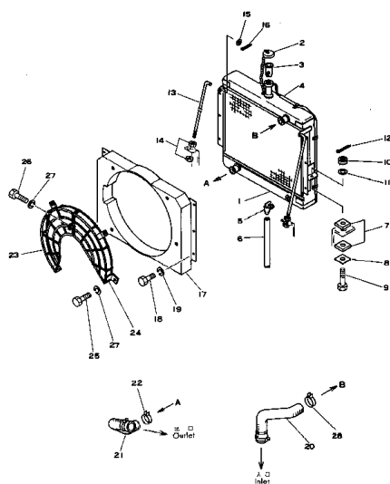
ラジエータ Fig. 112 RADIATOR
