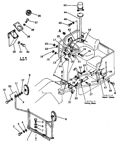
センタ エレクトリカル パーツ Fig. 142 CENTER ELECTRICAL PARTS
