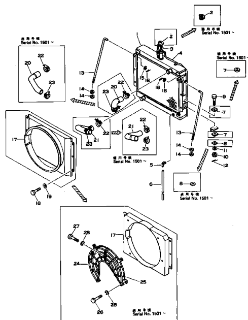
ラジエータ Fig. 121 RADIATOR
