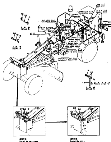
Fig. 132 WIRING (Serial No. 1003~1500)
