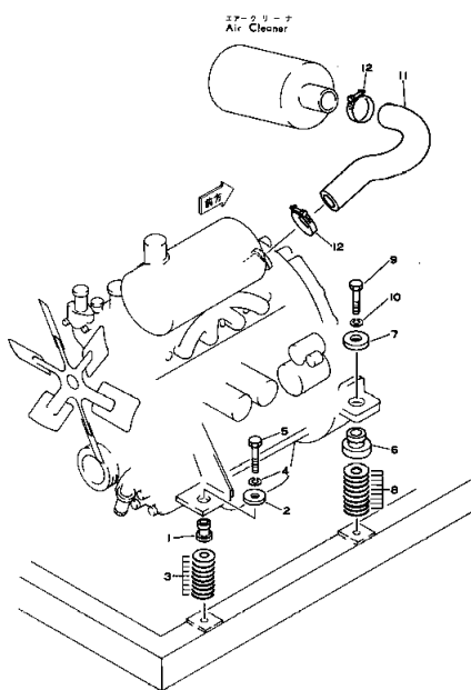
エンジン マウンティング パーツ (適用機種 Fig. 103 ENGINE MOUNTING PARTS (Serial No. 1501~))
