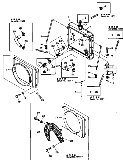
Fig. 121 ラジエータ RADIATOR
