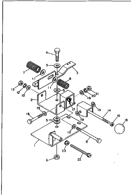
スロットルレバー組立 適用機種 FIG. 4501 THROTTLE LEVER ASS'Y (EG85BS SERIAL NO. 4501- )
