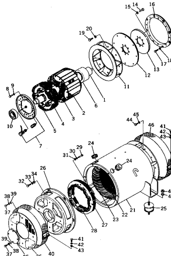
發電機組立圖 (EG85BS SERIAL NO. 4501- ) FIG. 1201 GENERATOR ASS'Y (EG85BS SERIAL NO. 4501- )
