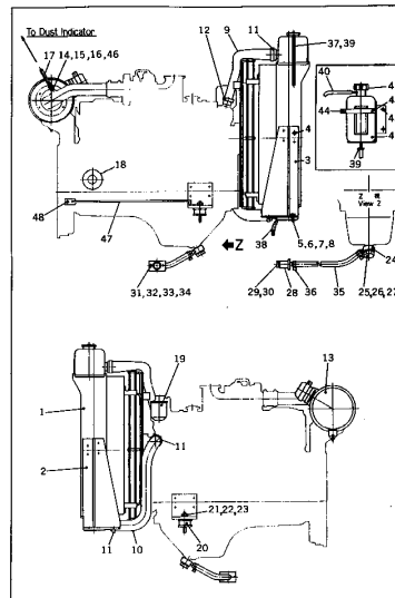
ラジエータ組立 適用機種 FIG. 3201 RADIATOR ASS'Y (EG85BS SERIAL NO. 4501-)
