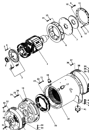
圖 1001 發電機組立 (EG85B 通用號碼 4001-UP) FIG. 1001 GENERATOR ASS'Y (EG85B SERIAL NO. 4001-UP) (EG85B SERIAL NO. 4001-UP)
