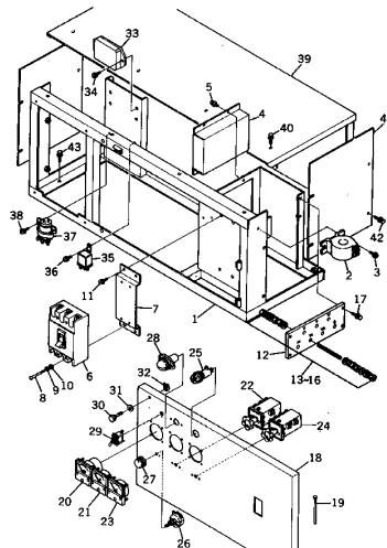
制 御 箱 組 立 FIG. 2001 CONTROL BOX ASS'Y (400/440V) 適用機種 (EG85 SERIAL NO. 4001- ) (EG85B SERIAL NO. 4001- )
