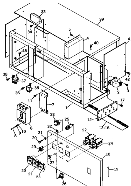
制 御 箱 組 立 FIG. 2101 CONTROL BOX ASS'Y (200/220V) 適用機種 (EG85 SERIAL NO. 4001-) (EG85B SERIAL NO. 4001-)
