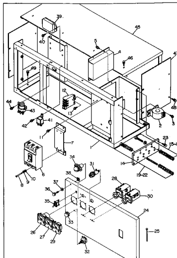
附 錄 圖 表 FIG. 2011 CONTROL BOX ASS'Y (200, 400/220, 440V) 適用 機種 (EG85 SERIAL NO. 4001- ) (EG85B SERIAL NO. 4001- )
