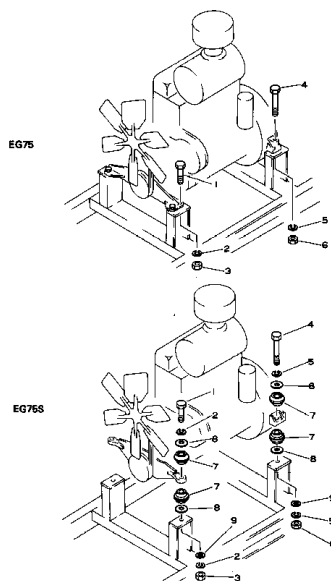
エンジン 取付 部品 Fig. 101 ENGINE MOUNTING PARTS
