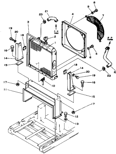
ラジオエータ および マウンティング ( 適用機種 EG75S Serial No. 1001~ ) Fig. 122 RADIATOR AND MOUNTING ( EG75S Serial No. 1001~ )
