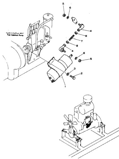
ソレノイド および マウンティング Fig. 111 SOLENOID AND MOUNTING
