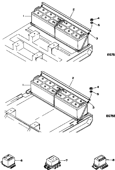
Fig. 141 バッテリー BATTERY
