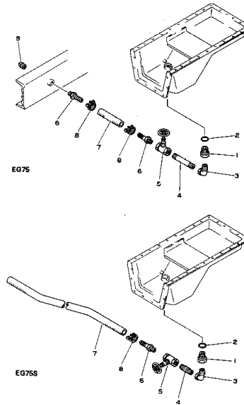
Fig. 161 オイル ドレン パイピング OIL DRAIN PIPING
