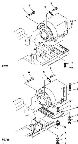
ジェネレータ 取付部品 Fig. 201 GENERATOR MOUNTING PARTS
