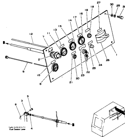
エンジン インストルメント パネル Fig. 145 ENGINE INSTRUMENT PANEL
