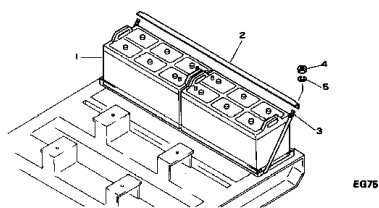
Fig. 141 バッテリー BATTERY
