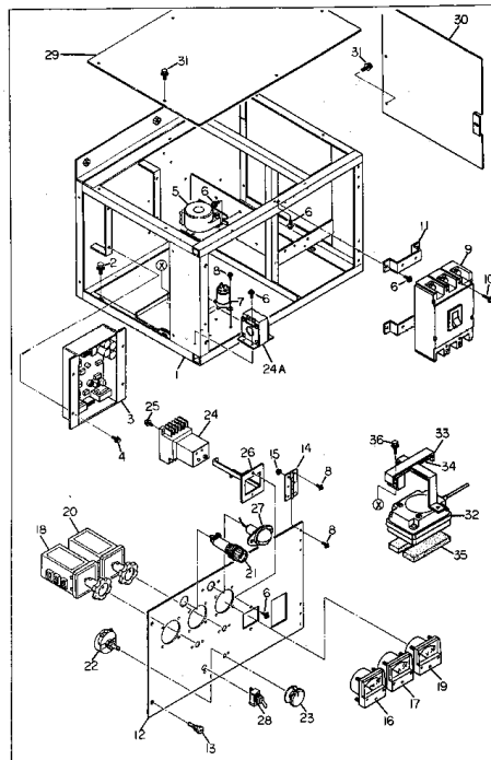
圖 2201 控制箱組立 FIG. 2201 CONTROL BOX ASS'Y (EG60BS)
