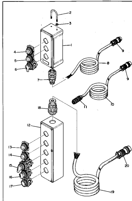
リモートコントロールボックス組立 FIG. 2251 REMOTE CONTROL BOX ASS'Y (EG60BS)
