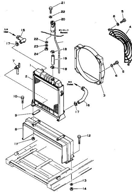
Fig. 122A ラジエータ および マウンティング (EG55S Serial No. 1087~) RADIATOR AND MOUNTING (EG55S Serial No. 1087~)
