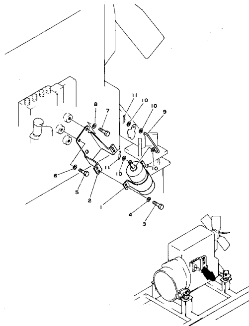
Fig. 111 ソレノイド および マウンティング (EG55 Serial No. 1001~1131) SOLENOID AND MOUNTING (EG55S Serial No. 1001~1086)
