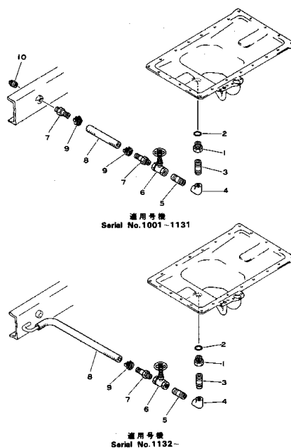
Fig. 161 オイル ドレン パイピング (適用機種 EG55 Serial No. 1001~)
