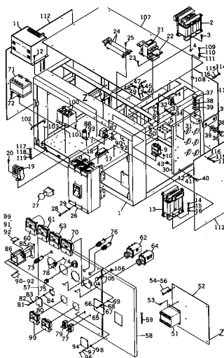
制御箱組立図 FIG. 2201 CONTROL BOX ASS'Y
