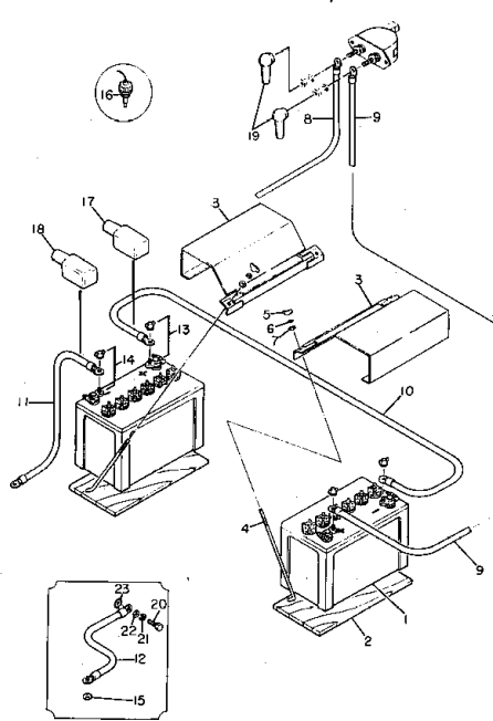
バッテリーアセンブリ FIG. 5201 BATTERY ASS'Y (EG40BS)
