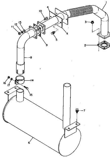
マフラー アセンブリ FIG. 6201 MUFFLER ASS'Y (EG40BS)
