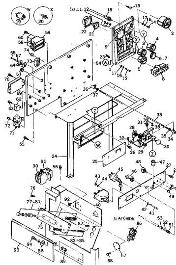
FIG. 4201 エンジン オペレーティングパネル アセンブリ (EG40BS)
