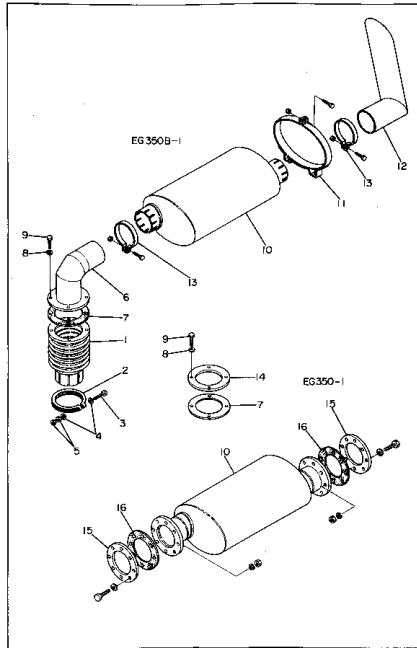
マフラー 組立 Fig. 6001 MUFFLER ASS'Y (EG350,350B)
