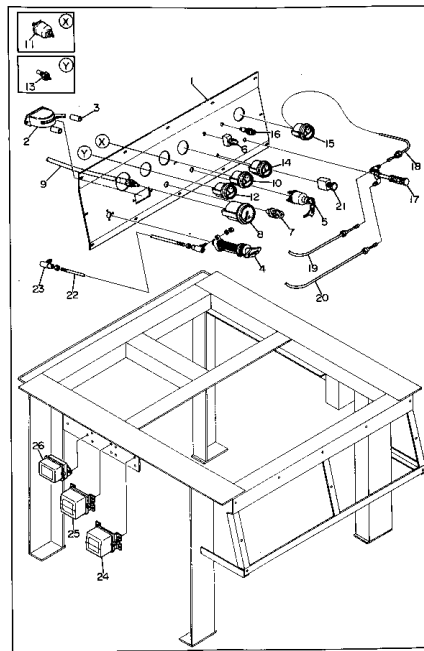
エンジン 操作盤 組立 Fig. 4001 ENGINE OPERATING PANEL ASS'Y (EG350,350B)
