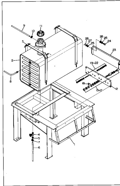
サポート レッグ および 燃料 タンク 組立 Fig. 7001 SUPPORT LEG AND FUEL TANK ASS'Y (EG350,350B)
