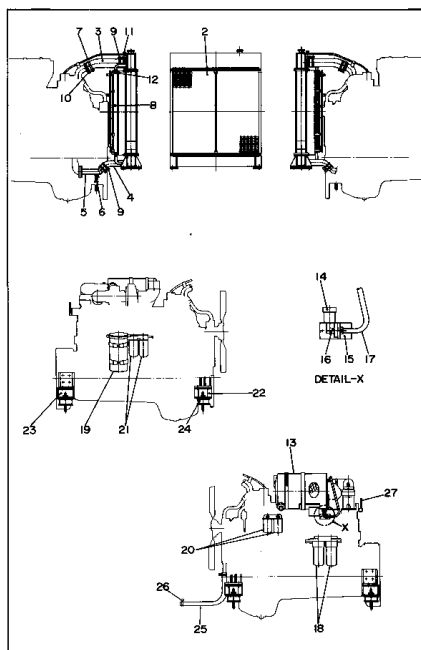
ラジエータ 組立 Fig.- 3001 RADIATOR ASS'Y (EG350,350B)
