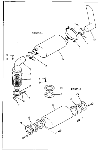
マフラー 組立 Fig. 8001 MUFFLER ASS'Y (EG350,350B)
