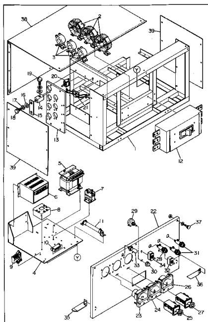
制 御 箱 組 立 Fig. 2001 CONTROL BOX ASS'Y (EG350,350B)
