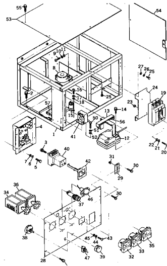
FIG. 2201 コントロール ボックスアセンブリ (EG33BS) FIG. 2201 CONTROL BOX ASS'Y (EG33BS)
