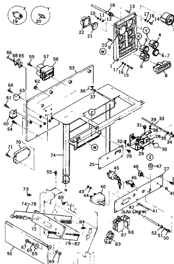
エンジン オペレーティング パネル アセンブリ FIG. 4201 ENGINE OPERATING PANEL ASS'Y (EG33BS)
