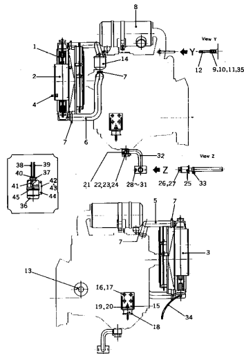
ラジエーター アセンブリ FIG. 3201 RADIATOR ASS'Y (EG33BS)
