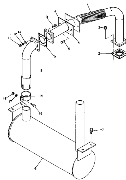
マフラー アセンブリ FIG. 6201 MUFFLER ASS'Y (EG33BS)
