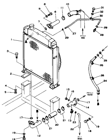
Fig. 121 ラジエーター および マウンティング RADIATOR AND MOUNTING
