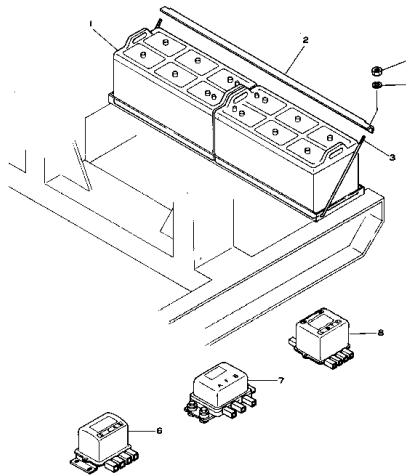
Fig. 141 バッテリー BATTERY
