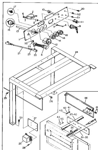
Fig. 4201 エンジン 操作盤 組立 ENGINE OPERATING PANEL ASS'Y (EG275BS)
