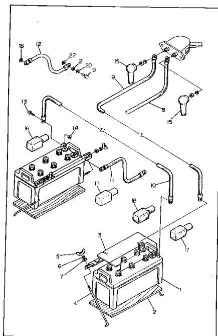
Fig. 5201 バッテリー 組立 BATTERY ASS'Y (EG275BS)
