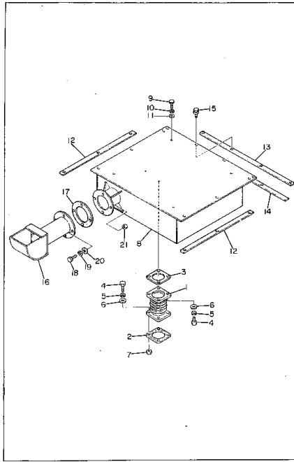
マフラー 組立 Fig. 6201 MUFFLER ASS'Y (EG275BS)
