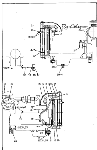
ラジエータ 組立 Fig. 3201 RADIATOR ASS'Y (EG275BS)
