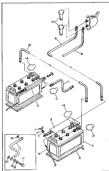
Fig. 5201 バッテリー 組立 BATTERY ASS'Y (EG220BS)
