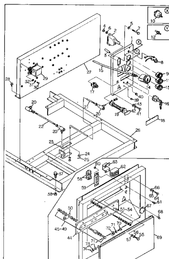
Fig. 4201 エンジン 操作盤 組立 ENGINE OPERATING PANEL ASS'Y (EG220BS)
