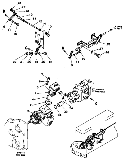
ガバナおよびスロットルレバー Fig. 111 GOVERNOR AND THROOFL LEVER
