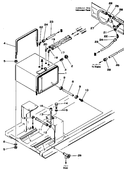
Fig. 131 フュエル タンク FUEL TANK
