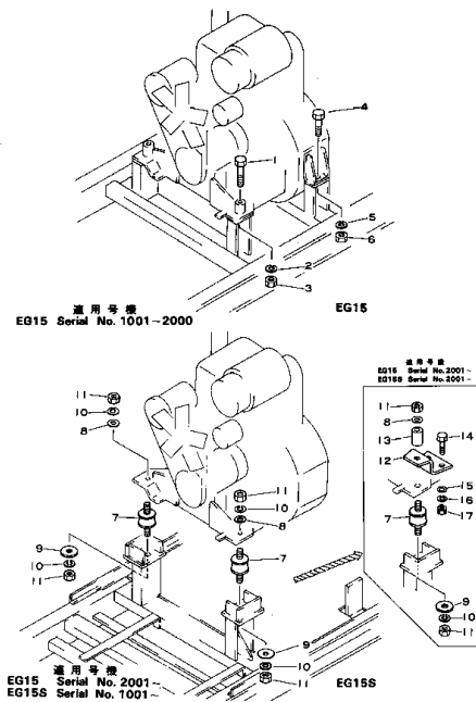
Fig. 101 エンジン 取付 部品 ENGINE MOUNTING PARTS
