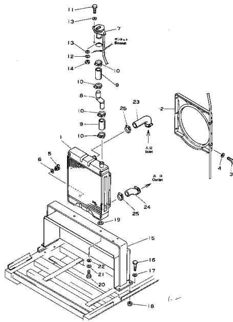
ラジエータ および マウンティング (EG15S 適用機種) Fig. 122 RADIATOR AND MOUNTING (EG15S Serial No. 1001~2000)
