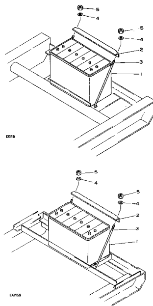
Fig. 141 バッテリー BATTERY
