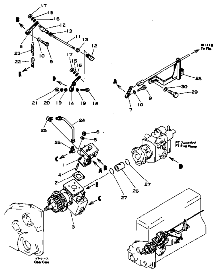
ガバナーおよびスロットルレバー Fig. 111 GOVERNOR AND THROTTLE LEVER
