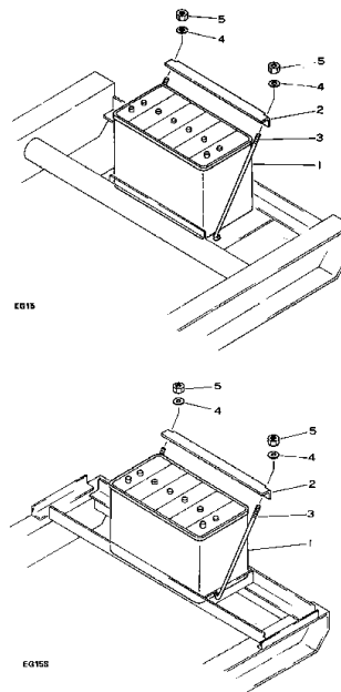
Fig. 141 バッテリー BATTERY
