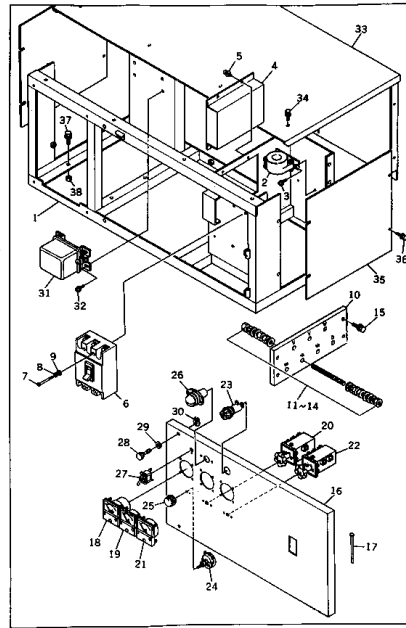
制御箱組立 FIG. 2101 CONTROL BOX ASS'Y (200/220V) 適用機種 海外向 (EG125 SERIAL NO. 4001-) (EXCEPT JAPAN) (EG125B SERIAL NO. 4001-)
