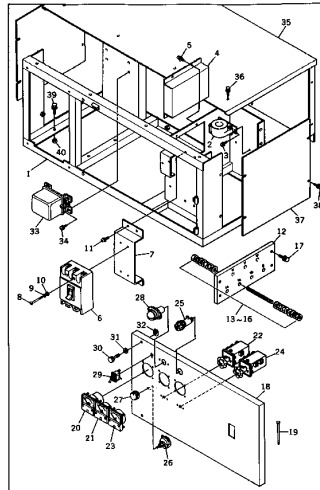
制 御 箱 組 立 図 FIG. 2001 CONTROL BOX ASS'Y (400/440V) 海 外 向 (EG125 SERIAL NO. 4001- ) (EXCEPT JAPAN) (EG125B SERIAL NO. 4001- )
