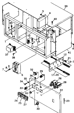
制 造 組 立 FIG. 2011 CONTROL BOX ASS'Y (200, 400/220, 440V) (EG125 SERIAL NO. 4001-) (EXCEPT JAPAN) (EG125B SERIAL NO. 4001-)
