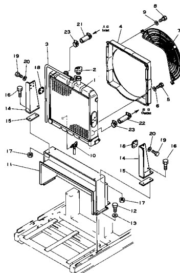
ラジエータ および マウンティング (適用 号機) Fig. 122 RADIATOR AND MOUNTING (EG100S Serial No. 1001~)
