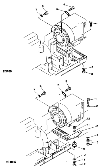
ジェネレータ 取付部品 Fig. 201 GENERATOR MOUNTING PARTS
