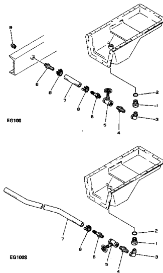
オイル ドレン パイピング Fig. 161 OIL DRAIN PIPING
