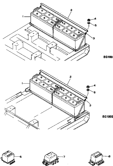
Fig. 141 バッテリ BATTERY
