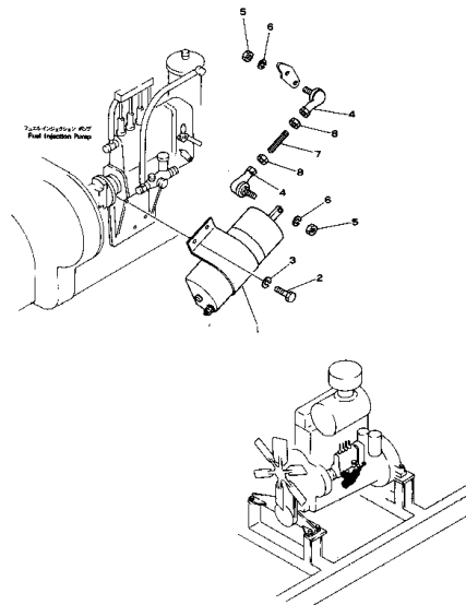
ソレノイド および マウンティング Fig. 111 SOLENOID AND MOUNTING
