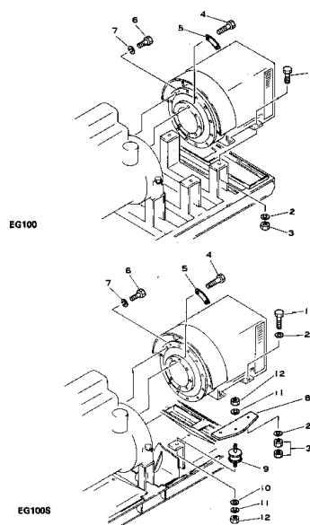
ジェネレータ 取付部品 Fig. 201 GENERATOR MOUNTING PARTS
