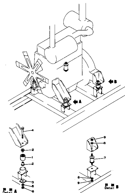
Fig. 101 エンジン取付部品 ENGINE MOUNTING PARTS
