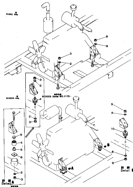
Fig. 101 エンジン取付部品 (EC50Z Serial No. 1001~3000) (EC50ZS Serial No. 1001~3000)
