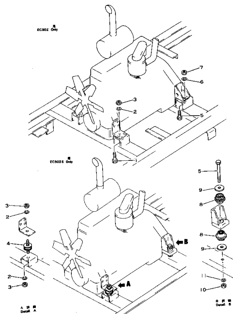
Fig. 101A エンジン取付部品 (EC50Z Serial No. 3001~) (EC50ZS Serial No. 3001~)
