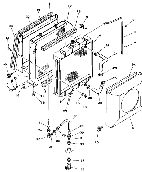
Fig. 121 ラジエーター および オイル クーラー (EC50Z Serial No. 1001~3000) (EC50ZS Serial No. 1001~3000)
