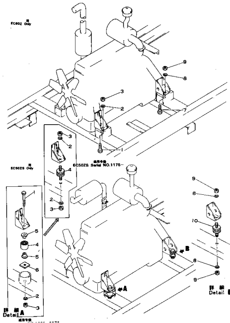
Fig. 101 エンジン取付部品 (ENGINE MOUNTING PARTS) (EC50Z Serial No. 1001~3000) (EC50ZS Serial No. 1001~3000)
