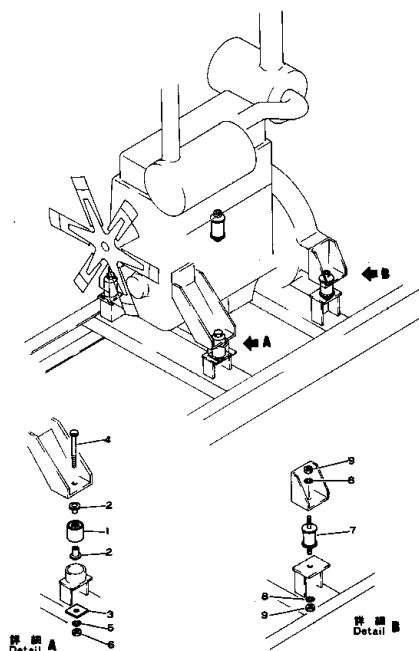
Fig. 101 エンジン 取付 取付部 ENGINE MOUNTING PARTS
