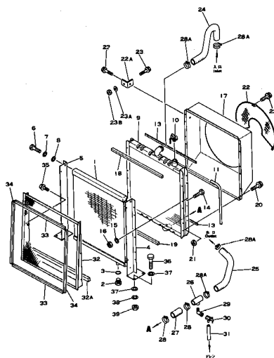
Fig. 121 RADIATOR
