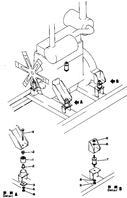
Fig. 101 エンジン 取付 取組 ENGINE MOUNTING PARTS
