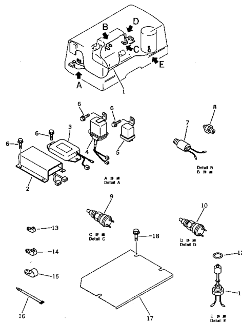
Fig. 151 エレキテリカル システム (EC35Z Serial No. 1001~1105) 海外用 (EC35ZS Serial No. 1001~1963) (Except Japan)
