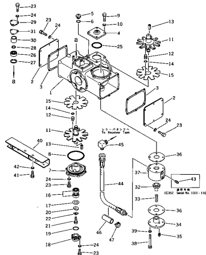
Fig. 201 CYLINDER
