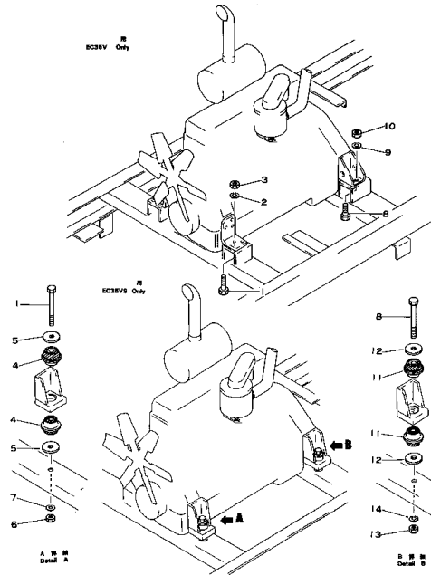
Fig. 101A エンジン 取付 部品 (EC35V Serial No. 3001~) (EC35VS Serial No. 3001~)
