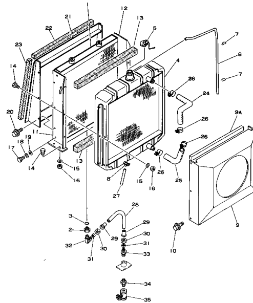
Fig. 121 ラジエータ および オイル クーラ (EC35V Serial No. 1001~3000) (EC35VS Serial No. 1001~3000)
