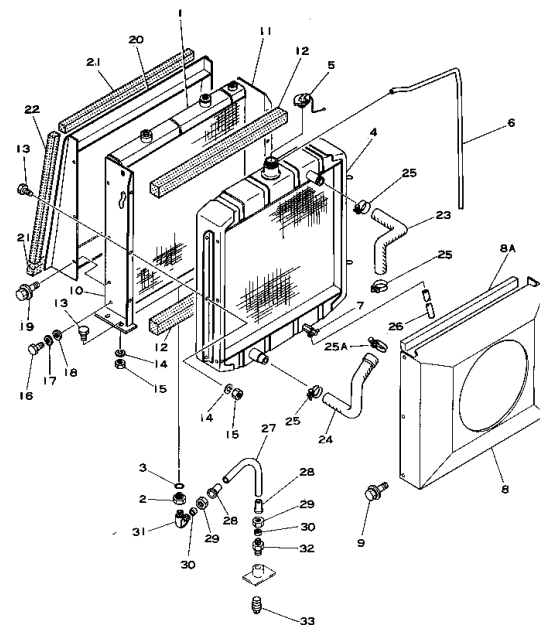
Fig. 121A ラジエータ および オイル クーラ (EC35V Serial No. 3001~3442) (EC35VS Serial No. 3001~3762)
