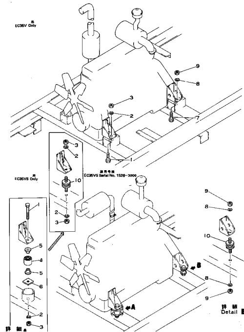
Fig. 101 エンジン 取付 部品 (EC35V Serial No. 1001~3000) (EC35VS Serial No. 1001~3000)
