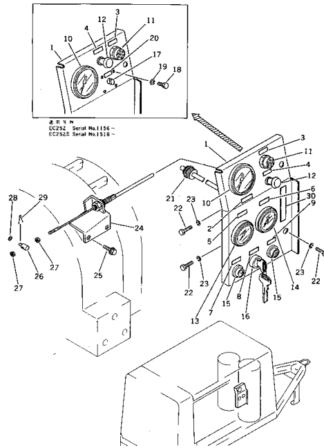
Fig. 145 インストルメント パネル INSTRUMENT PANEL
