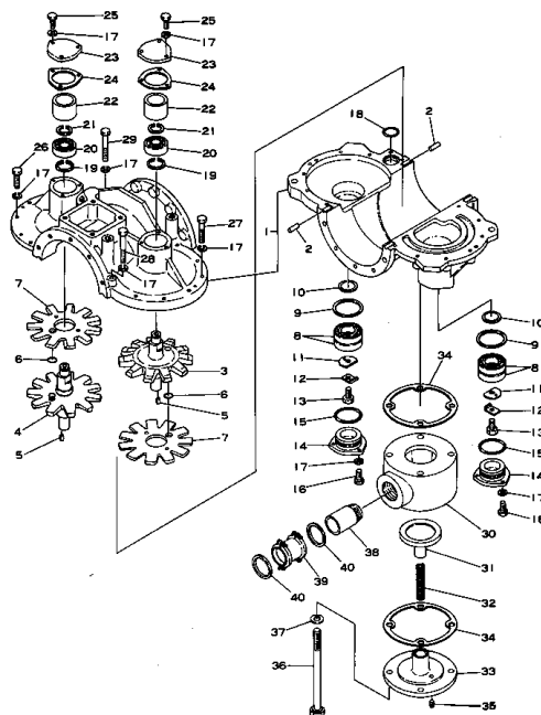
Fig. 201 シリンダ CYLINDER
