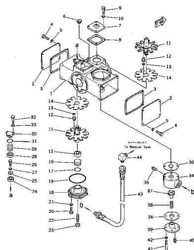
Fig. 201 CYLINDER
