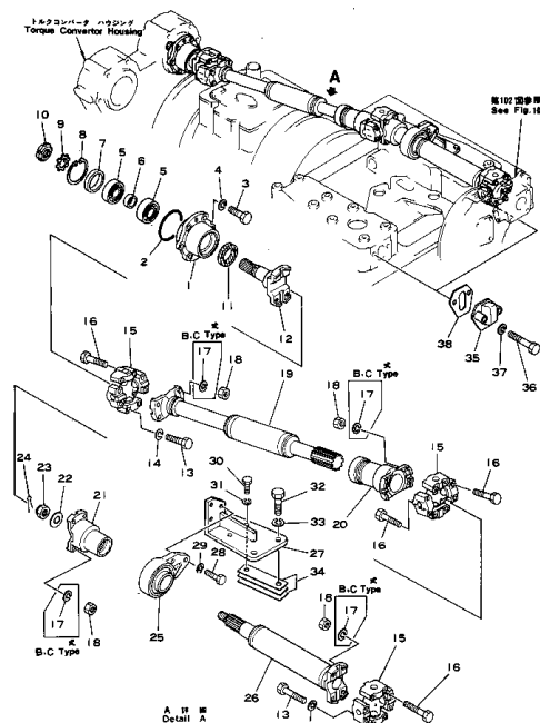
P.T.O. シャフト Fig. 101 P.T.O. SHAFT
