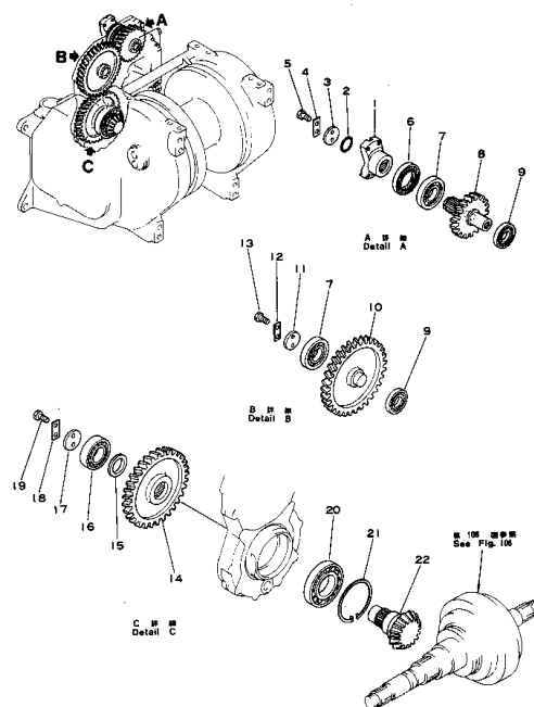
トランスファー ギヤー Fig. 103 TRANSFER GEAR
