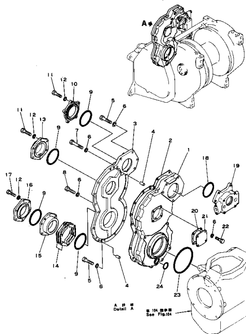
トランスファー ケース Fig. 102 TRANSFER CASE
