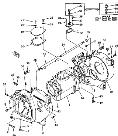
ギヤ ケース Fig. 104 GEAR CASE
