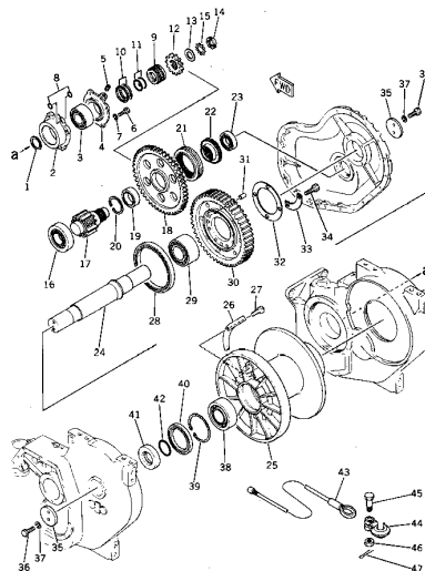
Fig. 207 ギヤー および ドラム GEAR AND DRUM
