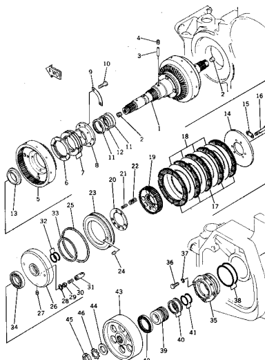
Fig. 206 クラッチ、および プレーキ ドラム CLUTCH AND BRAKE DRUM
