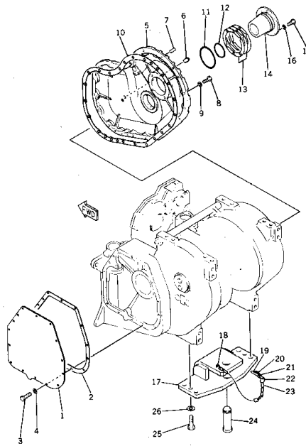
Fig. 205 ケース カバー および ヒッチ CASE COVER AND HITCH
