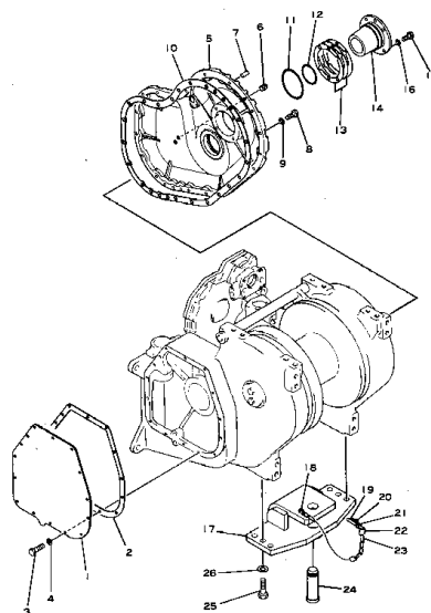
ケース カバー および ヒッチ Fig.105 CASE COVER AND HITCH
