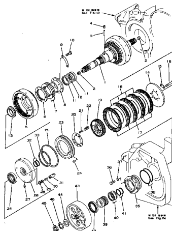
クラッチ および ブレーキ ドラム Fig.106 CLUTCH AND BRAKE DRUM
