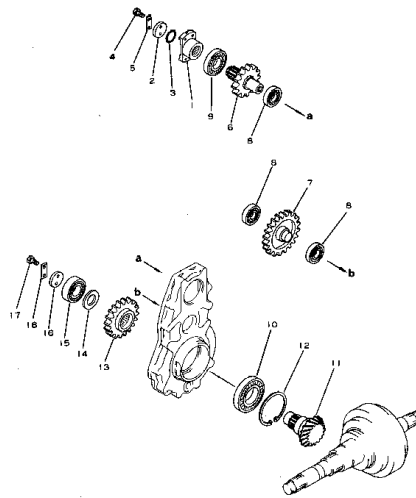
トランスファー ギヤ Fig. 103 TRANSFER GEAR
