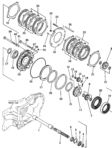
ウインディング シフト クラッチ (1) Fig. 202 WINDING SHIFT CLUTCH (1)
