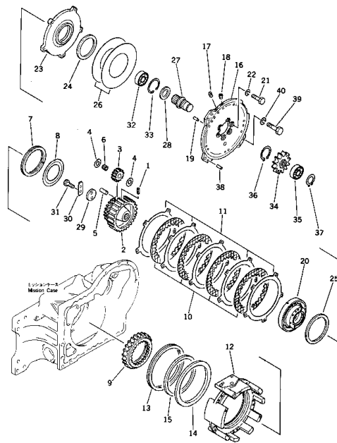
ウインディング シフト クラッチ Fig. 203 WINDING SHIFT CLUTCH (2)
