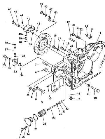
Fig. 201 ミッション ケース MISSION CASE
