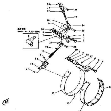
ブレーキ バンド Fig. 106 BRAKE BAND
