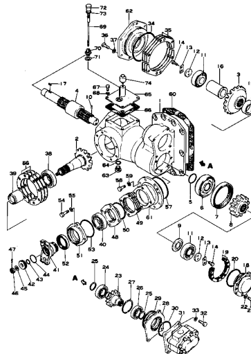
インプット シャフト および ハイドロリック ポンプ Fig. 102 INPUT SHAFT AND HYDRAULIC PUMP
