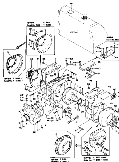
ケース および カバー Fig.106 CASE AND COVER
