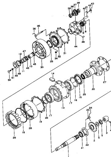
ドラム, 左 (適用機種) Fig. 121 DRUM, L.H. (Serial No. 1001~1999)
