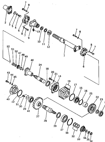
インプットシャフトおよびギヤ (適用機種) Fig. 111A INPUT SHAFT AND GEAR (Serial No. 2001~)
