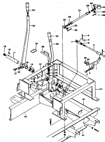
Fig. 1.95 コントロールレバーおよび車体改善部品 CONTROL LEVER AND MODIFIED CHASSIS PARTS (適用年表 Serial No. 1001 ~ 1999)
