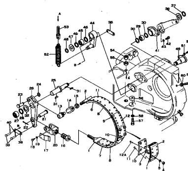
Fig. 104 BRAKE
