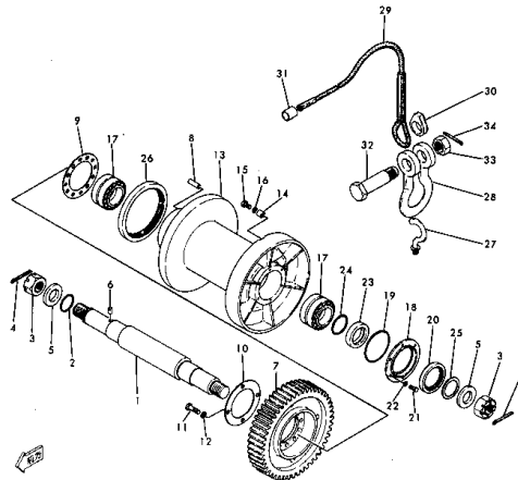
ケーブルドラム および シャフト Fig. 106 CABLE DRUM AND SHAFT, DWC060-1A, 1B, 1C, 1D, 1E
