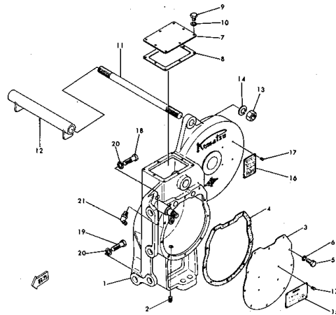
サイド フレーム, 左 Fig. 104 SIDE FRAME, L.H., DWC060-1B, 1D
