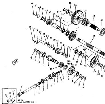
Fig. 101 POWER LINE, DWC060-1A, 1B, 1C, 1D, 1E
