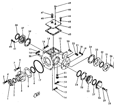
Fig. 102 CASE, DWC060-1A, 1B, 1C, 1D, 1E
