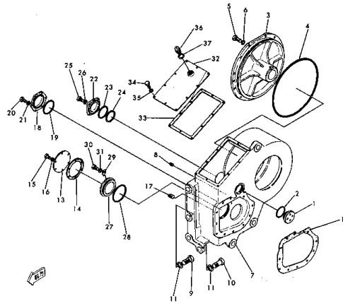
サイド フレーム, 右 Fig. 105 SIDE FRAME, R.H., DWC060-1A, 1B, 1C, 1D, 1E
