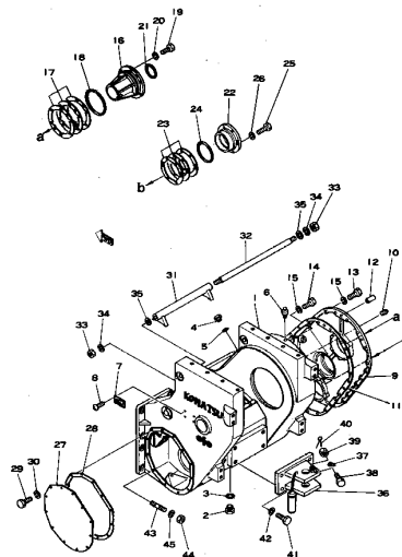
ケースおよびドロワー Fig. 101 CASE AND DRAWBAR
