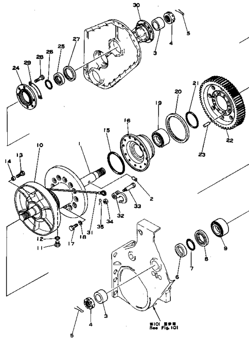
ドラム (D50A,P,S 適用機種) Fig. 105 DRUM (D50A,P,S Serial No. 59001~64999)
