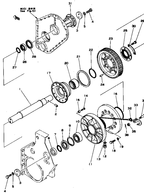
ドラム / 適用機種 Fig. 105A DRUM(D50A,P.S Serial No. 65001~)
