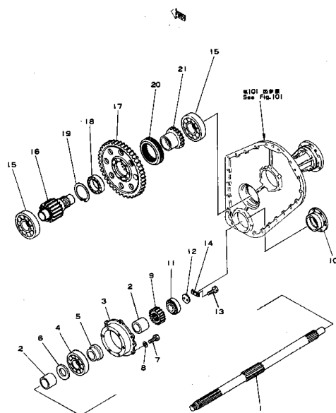
ギヤー( 適用機種 Fig. 104A GEAR(D50A,P,S Serial No. 65001~)
