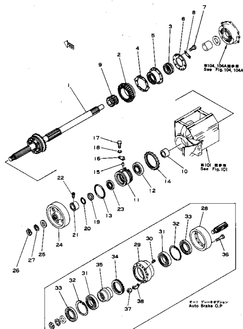
P.T.O. シャフト および ブレーキ ドラム Fig. 103 P.T.O. SHAFT AND BRAKE DRUM
