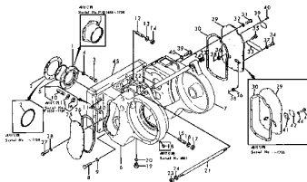
ケース および ハイドロリック タンク ブラケット Fig. 101A CASE AND HYDRAULIC TANK BRACKET (適用機番 Serial No.1001～1756)
