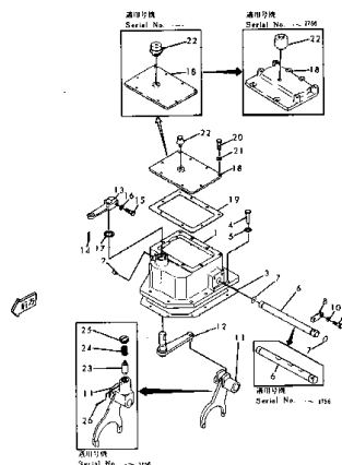
Fig. 104 フォーク および ケース (適用号機 (16001)~1756) FORK AND CASE (Serial No. (16001)~1756)
