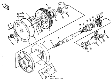
ドラム および ドライブ ギヤ (適用号 16001~1756) Fig. 105 DRUM AND DRIVE GEAR (Serial No. (16001)~1756)
