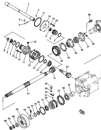
Fig. 202 P.T.O. シャフト、ギヤ、ブレーキ ドラム P.T.O. SHAFT AND BRAKE DRUM
