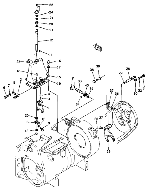
Fig. 206 シフト フォーク SHIFT FORK
