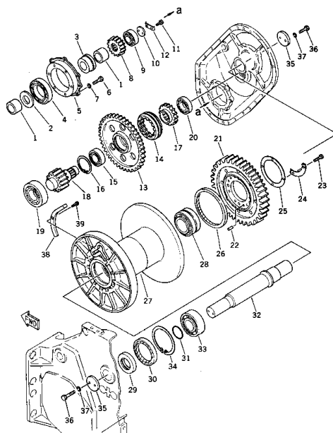
Fig. 203 ギヤー および ドラム GEAR AND DRUM
