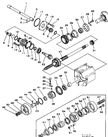
Fig. 102 P.T.O. SHAFT AND BRAKE DRUM P.T.O. シャフト、ブレーキドラム
